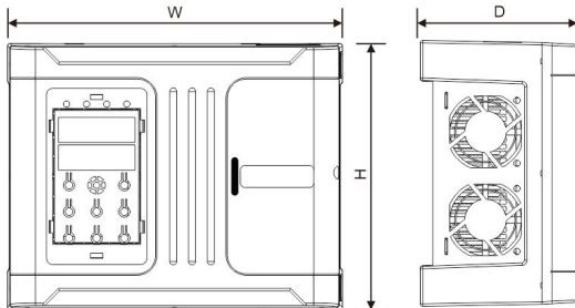
图 2-5-1 产品外型尺寸(单位: mm)
